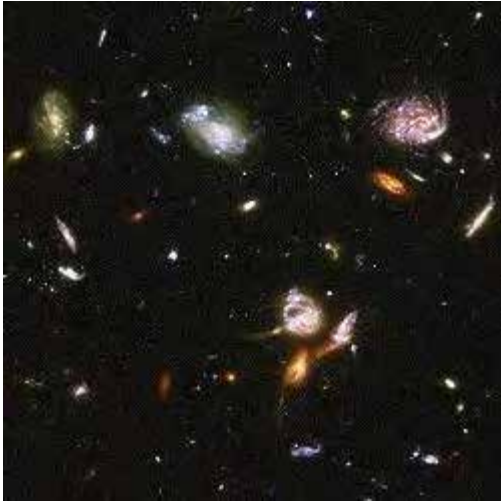
Figuur 2: Sterrenstelsels op een afstand van 12,7 lichtjaren = 12,7 \times 9,4 = 119 biljoen km.
